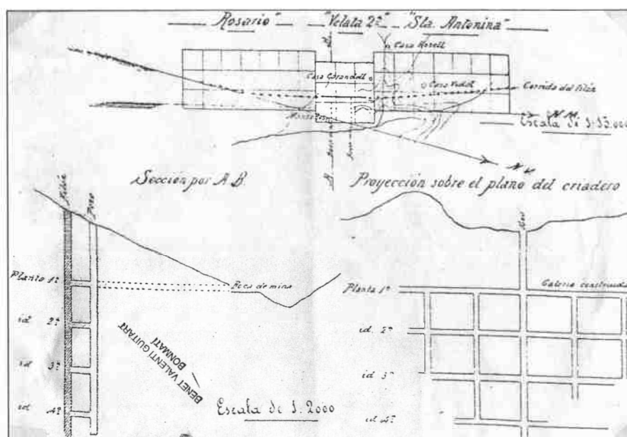
Plano del 1911 de les mines de plom "Velata Ila", "Santa Antonina" i "Rosario", de 51 pertinences o hectàrees situades a Sant Julià del Llor.
